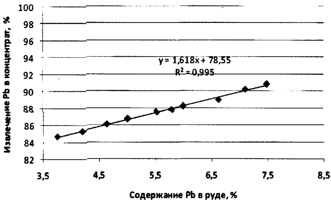
Рис. 1. Зависимость извлечения свинца от содержания его в руде
