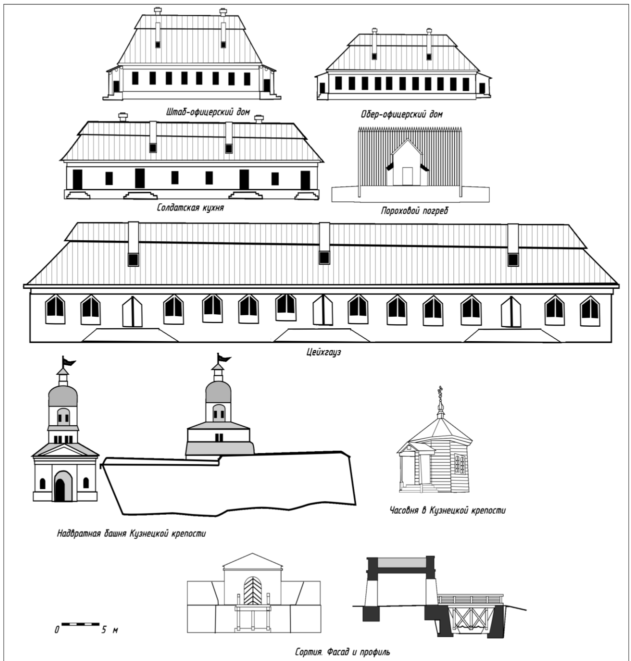
Рисунок А.2 – Прорисовка фасадов и общего вида строений Кузнецкой крепости. Слева направо и сверху вниз: штаб-офицерский дом, обер-офицерский дом, солдатская кухня, пороховой погреб, цейхгауз, надвратная башня (фасад и вид сбоку), часовня (прорисовка фотографии), сортия (фасад и профиль). (По материалам сайта «Кузнецкая крепость»)
