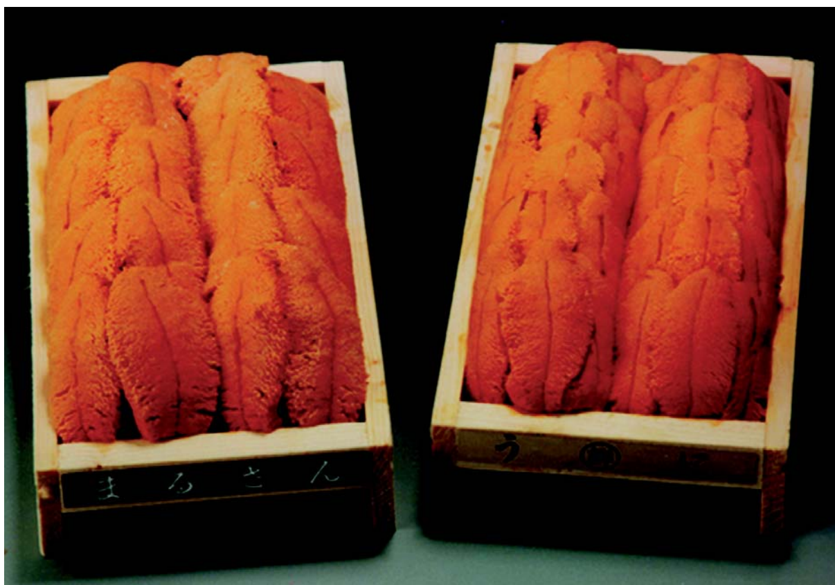
Рис. 8. Типичный способ укладки икры морских ежей на деревянные лотки для оптовой продажи
