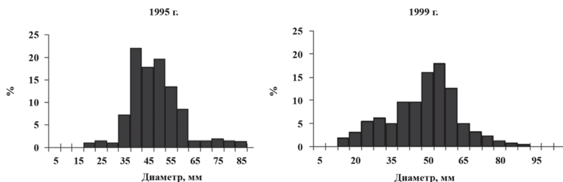
Рис. 4.3.4. Размерно-частотное распределение многоиглового морского ежа в районе б. Вилучинской на глубине 2–7 м в 1995 и 1999 гг.
