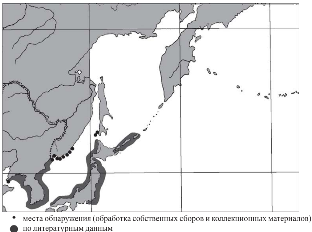
Рис. 2.1.5. Географическое распространение Mesocentrotus nudus
