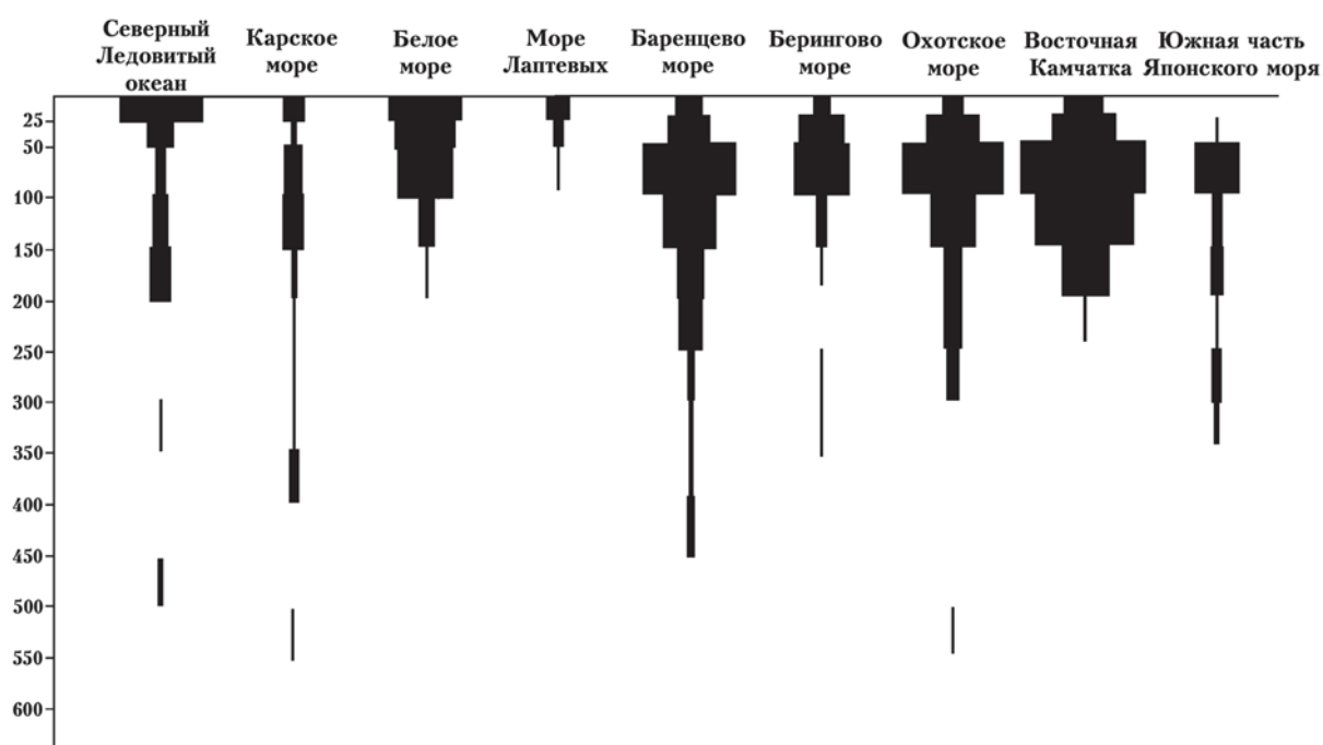
Рис. 3.1.1. Батиметрическое распределение Strongylocentrotus pallidus в морях России. По вертикали — глубина, м. Ширина столбиков соответствует количеству находок вида в соответствующем интервале глубин
