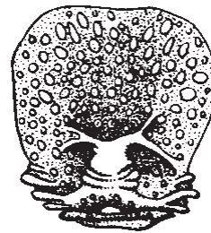
Рис. 1.1.7. Створка трифильной педицеллярии (по: Иванов и др., 1981)
