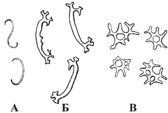
Рис. 1.1.11. Спикюлы в толще глобиферной педицеллярии (А), стенки амбулакральной ножки (Б) и стенках жабр (В) (по: Иванов и др., 1981)
