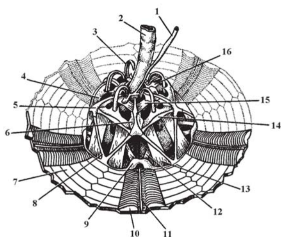
Рис. 1.1.13. Мускулатура аристотелева фонаря и органы, концентрирующиеся вокруг него. Вид изнутри (по: Иванов и др., 1981): 1 — осевой комплекс, впадающий в окологлоточный сосуд амбулакальной системы, 2 — пищевод, 3 — аборальный крючок зуба, 4 — аборальный край пирамидки (эпифизы), 5 — дужка, 6 — скобка, 7 — интеррадиальные пластинки скорлупы, 8 — мышечный пучок, протянутый между дужкой и оральным краем скорлупы, 9 — аурикулы, 10 — ампулы амбулакальных ножек, 11 — радиальный амбулакальный сосуд, 12 — ретракторы зуба, 13 — протракторы зуба, 14 — связки между концами дужек, 15 — мышцы, сокращением которых опускается аристотелев фонарь, 16 — полиев пузырь, связанный с окологлоточным кольцевым амбулакальным сосудом
